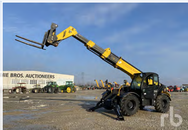
HAULOTTE HTL4017
